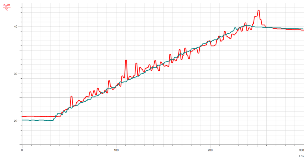
Abb. 21: zwei Diagramme zum Vergleich - Verbrennungskalorimeter III rot: nur Ringrührer verwendet, grün: Propellerrührer + Ringrührer verwendet
