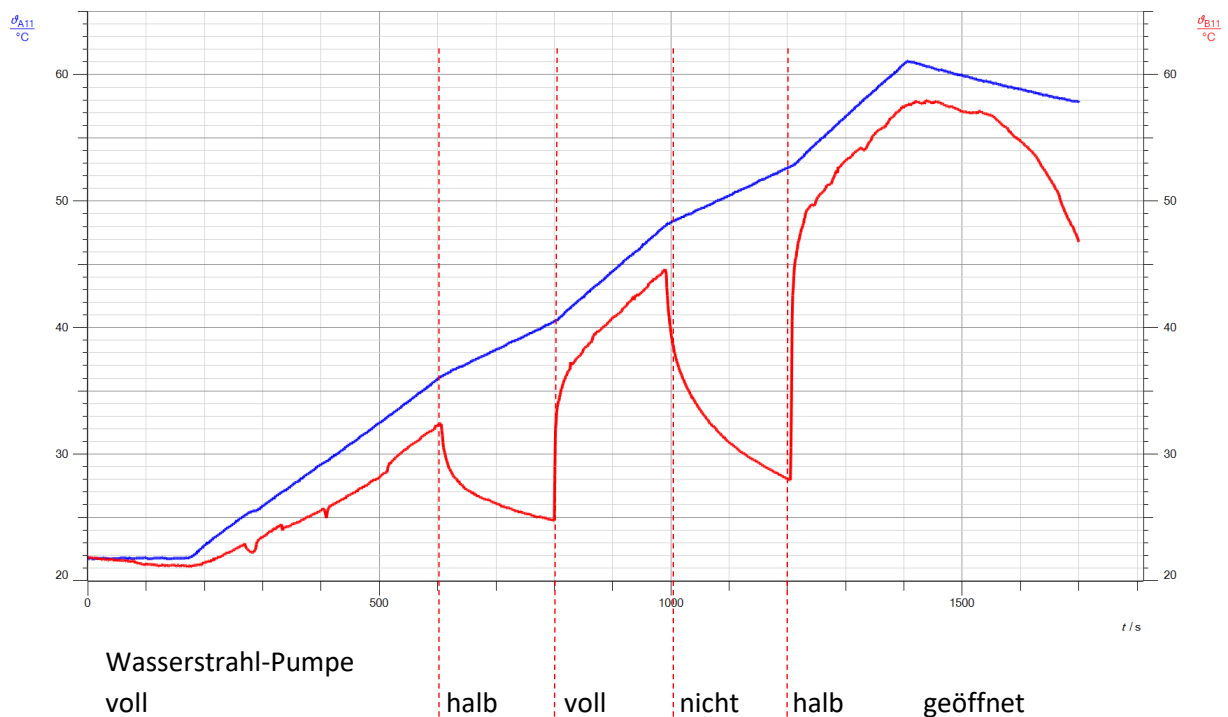
Abbildung 19: Veränderung der Abgas-Temperatur bei Veränderung des Unterdrucks der Pumpe (blau: Wassertemperatur, rot: Abgastemperatur)
