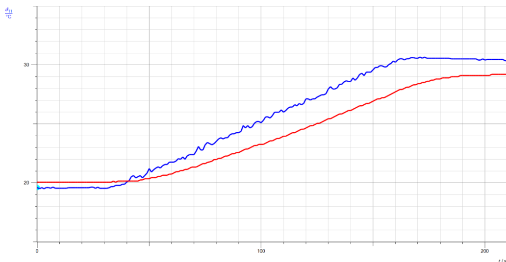
Abbildung 18: Verbrennungsenthalpie von Autogas Temperatur/Zeit-Diagramm (blau: Wassertemperatur, rot: Abgastemperatur)
